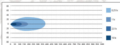
W-LIGHT MINI 161 mm. Kaugtulede paar
