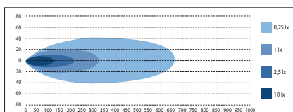
X-VISION OPTIMA 8 404 mm
