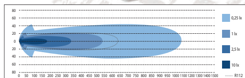
W-LIGHT BOOSTER 7 Double up – kahe võimsusega
