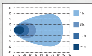
BULLPRO CENTUM 6000 K 100 W
