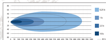
SEEKER ULTIMA 20 464 mm. Double up – kahe võimsusega
