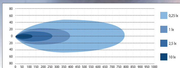
SEEKER CYCLOPS Kumer klaas, parktulega
